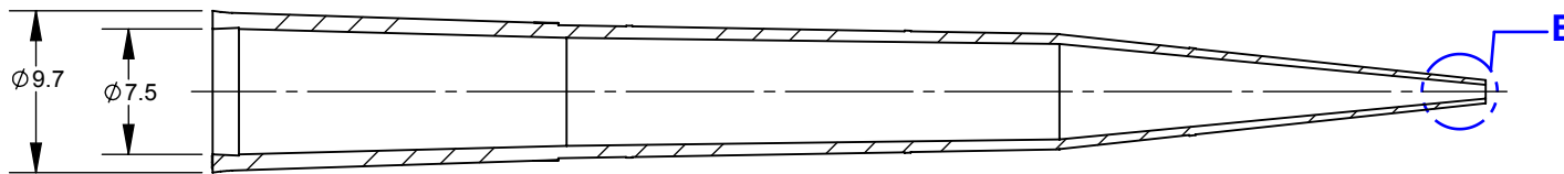
SECTION A-A
